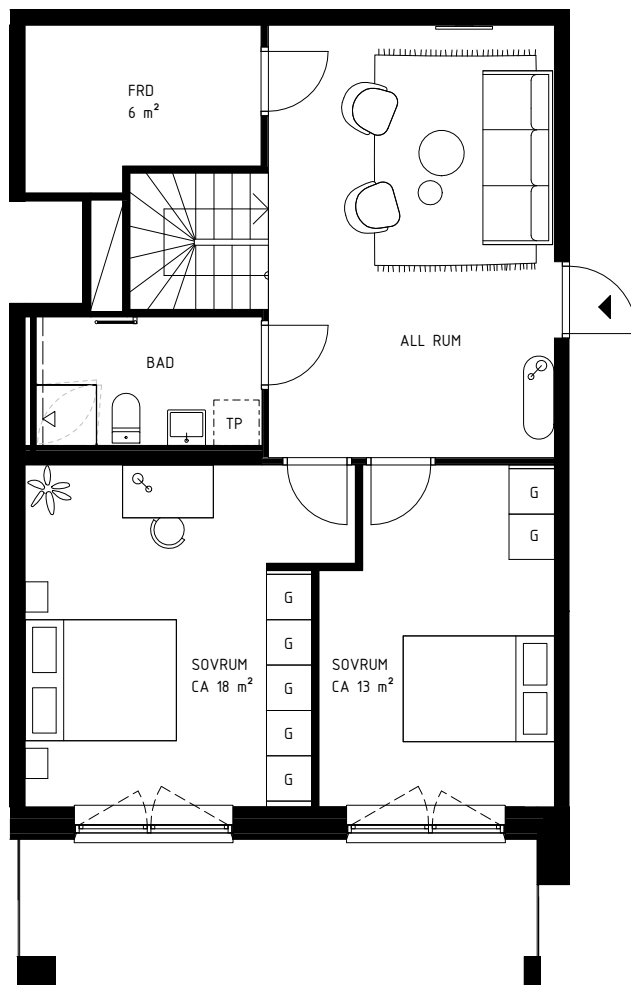
ÖVRE PLAN 70 m 2
