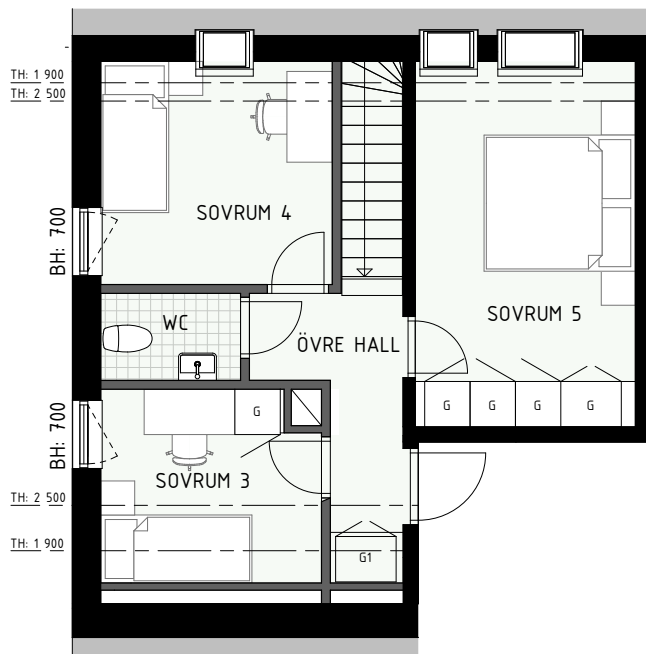
ÖVRE PLAN
